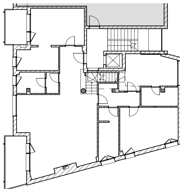
PIANTA PIANO SESTO - STATO DI FATTO
