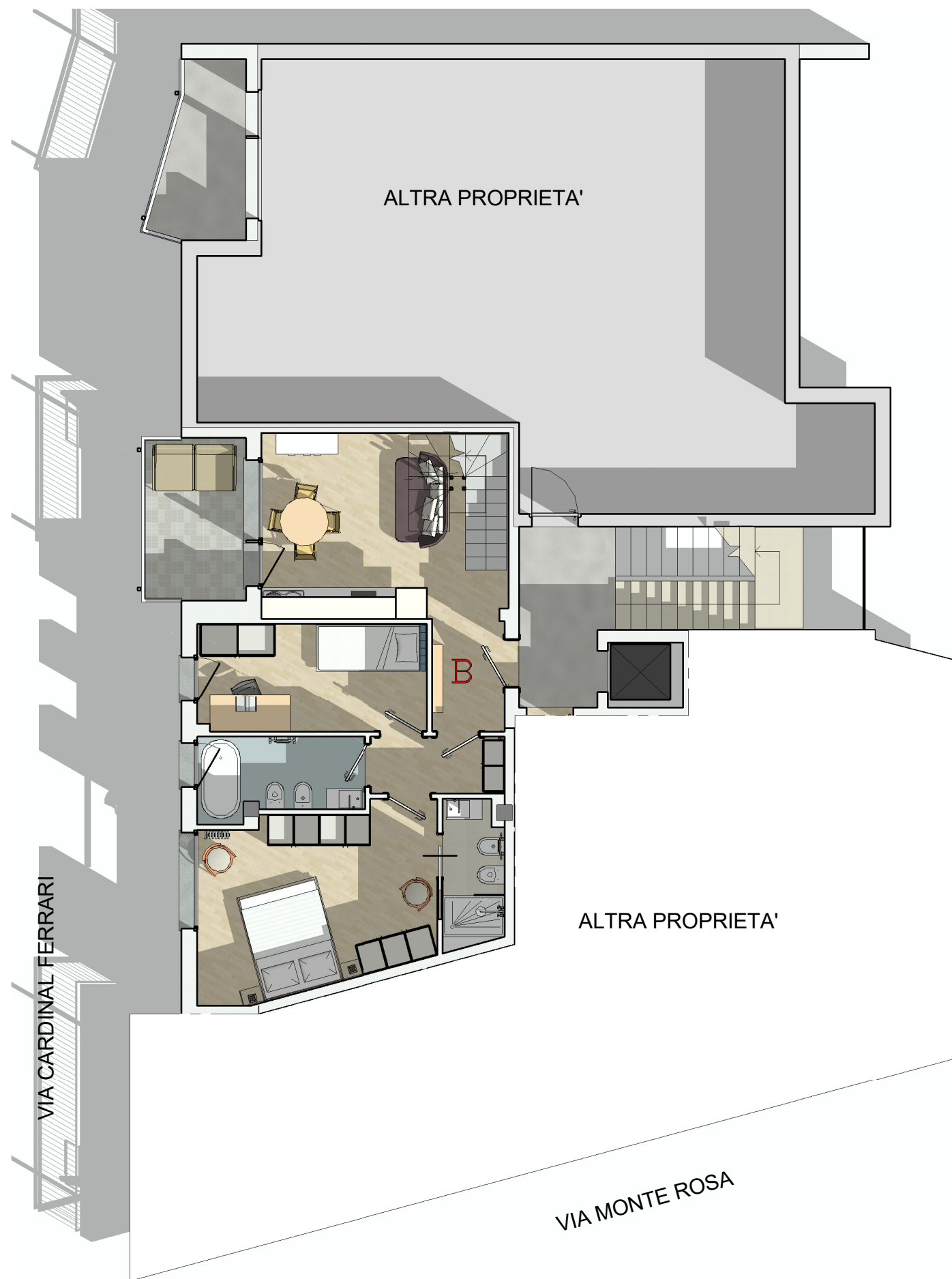
PIANTA PIANO SESTO - Appartamento B
